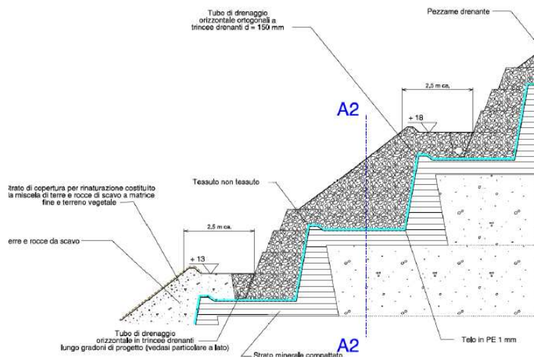
Particolare scarpata esterna
